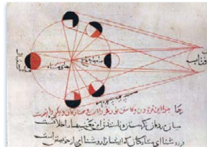
Ойнинг тўлиш босқичлари (Беруний чизмаси)
